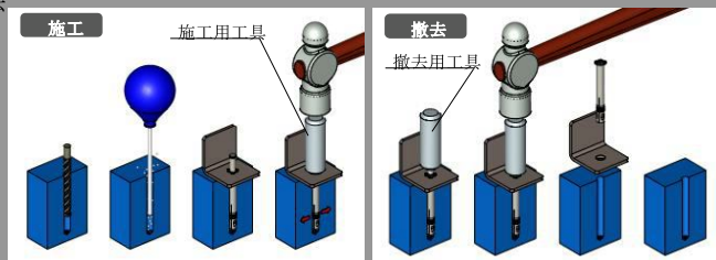
①下穴をあける②穴を清掃する ③挿入 ④芯金を打込む ①工具をセット②工具を叩く③アンカーを抜④完了
